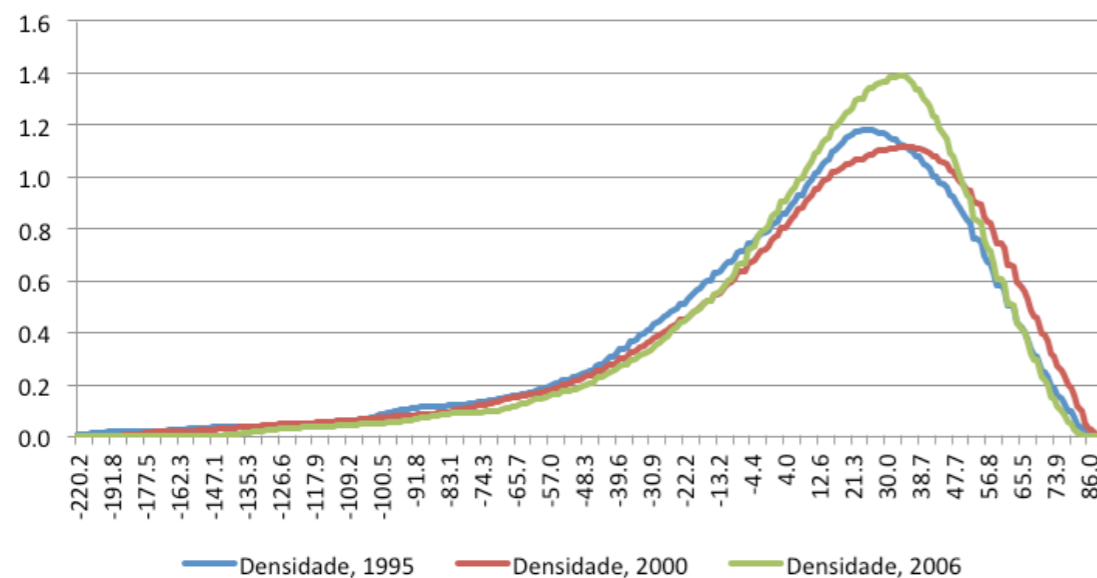
DENSIDADES DE PROBABILIDADE PARA A TAXA DE POUPANÇA
